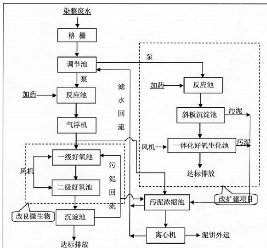
图 3.4-5 污水站废水处理工艺流程图
