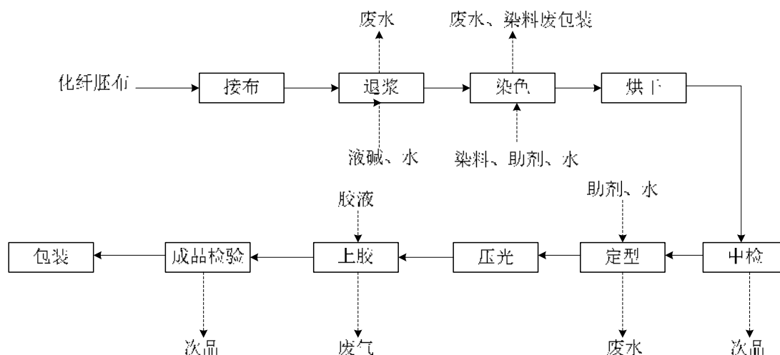
图 3.4-1 长纤染布生产工艺流程图
