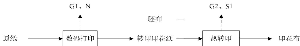
图 3.4-3 数码印刷生产线工艺流程图
