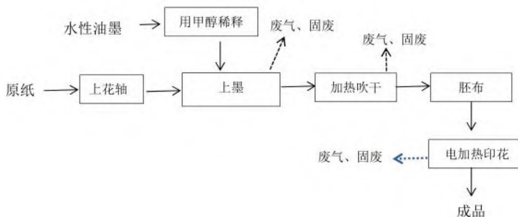
3.4-2 滚筒热转印生产线工艺流程图
