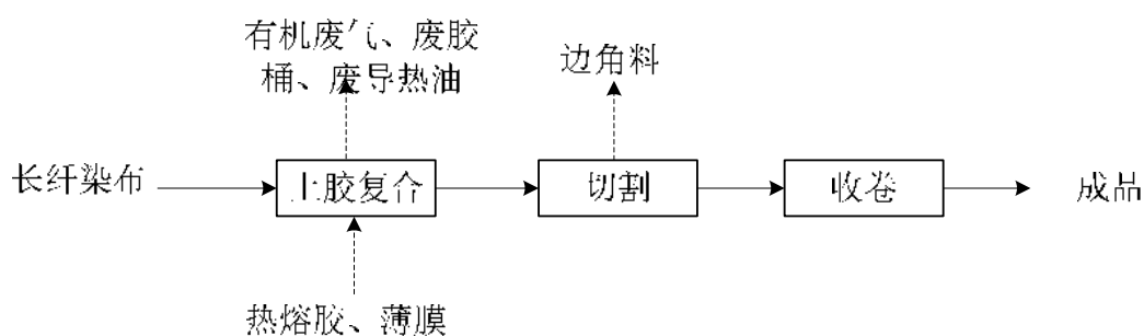
图 3.4-4 长纤染布技术改造生产线工艺流程图
